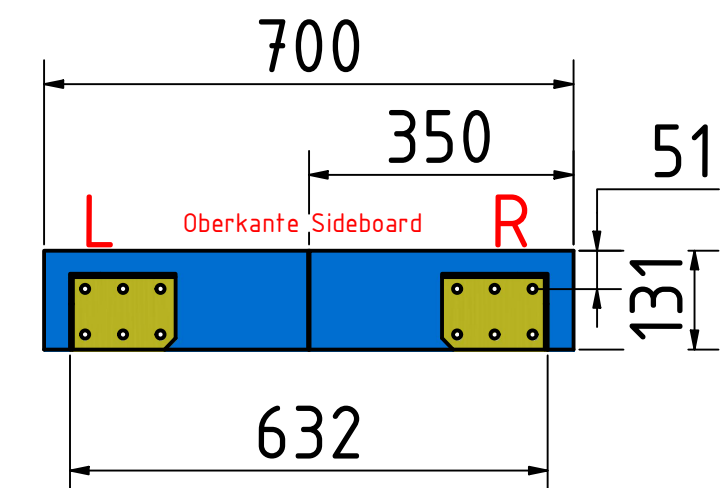
Bohrschablone 357_70-50-30
